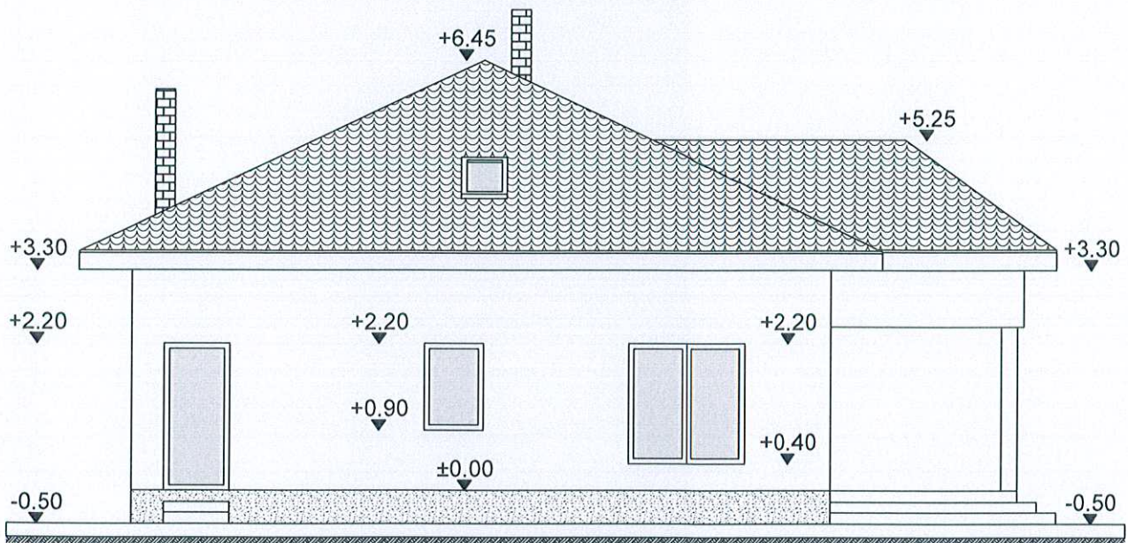
FAȚADA LATERALĂ-STÂNGA sc.1:100
