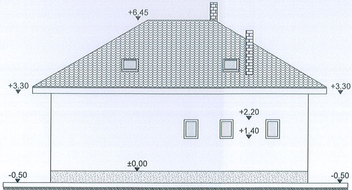
FAȚADA POSTERIOARĂ sc.1:100
