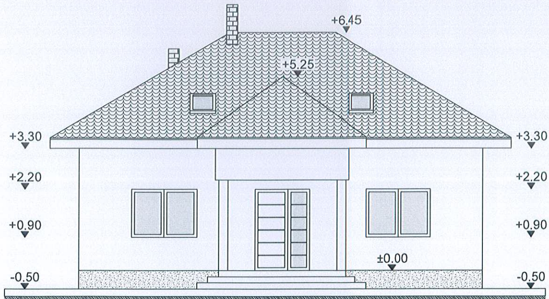
FAȚADA PRINCIPALĂ sc.1:100
