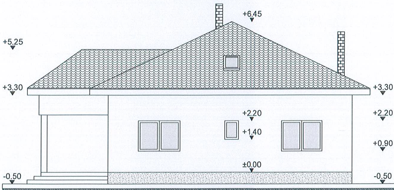
FAȚADA LATERALĂ-DREAPTA sc.1:100
