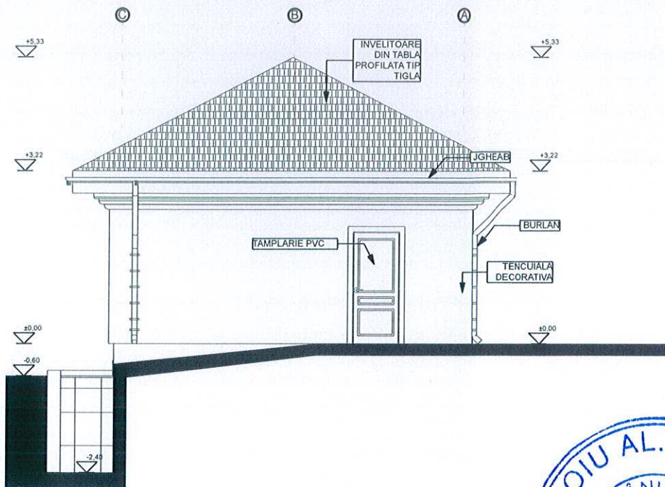
FATADA LAT. STANGA SC. 1:100
