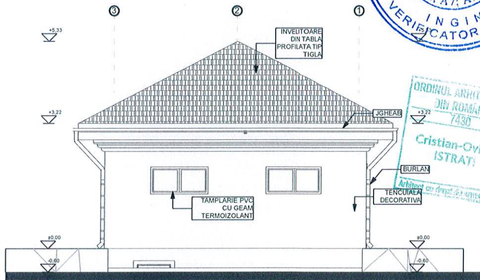
FATADA POSTERIOARA SC. 1:100
