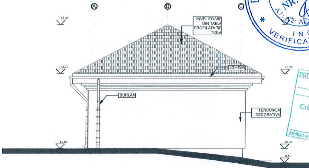
FATADA LAT. STANGA SC. 1:100
