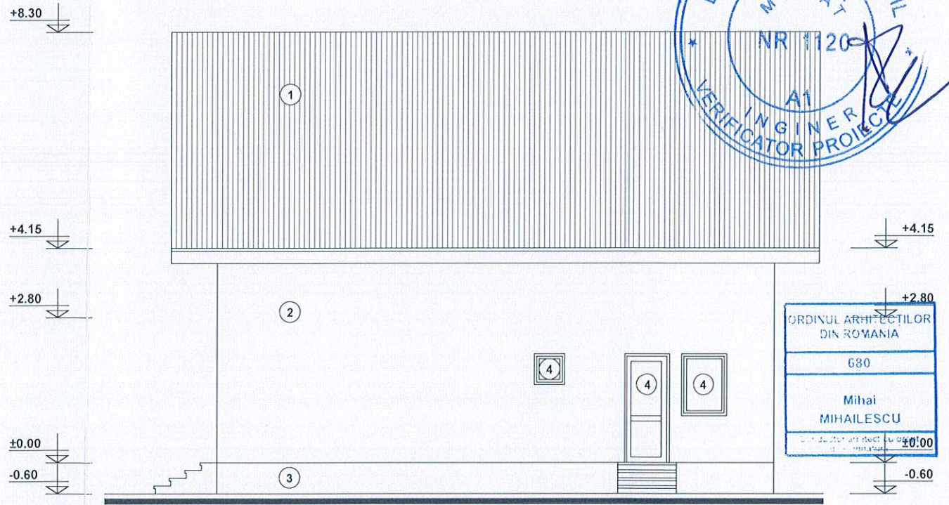
FATADA LATERALA DREAPTA Scara 1:100
