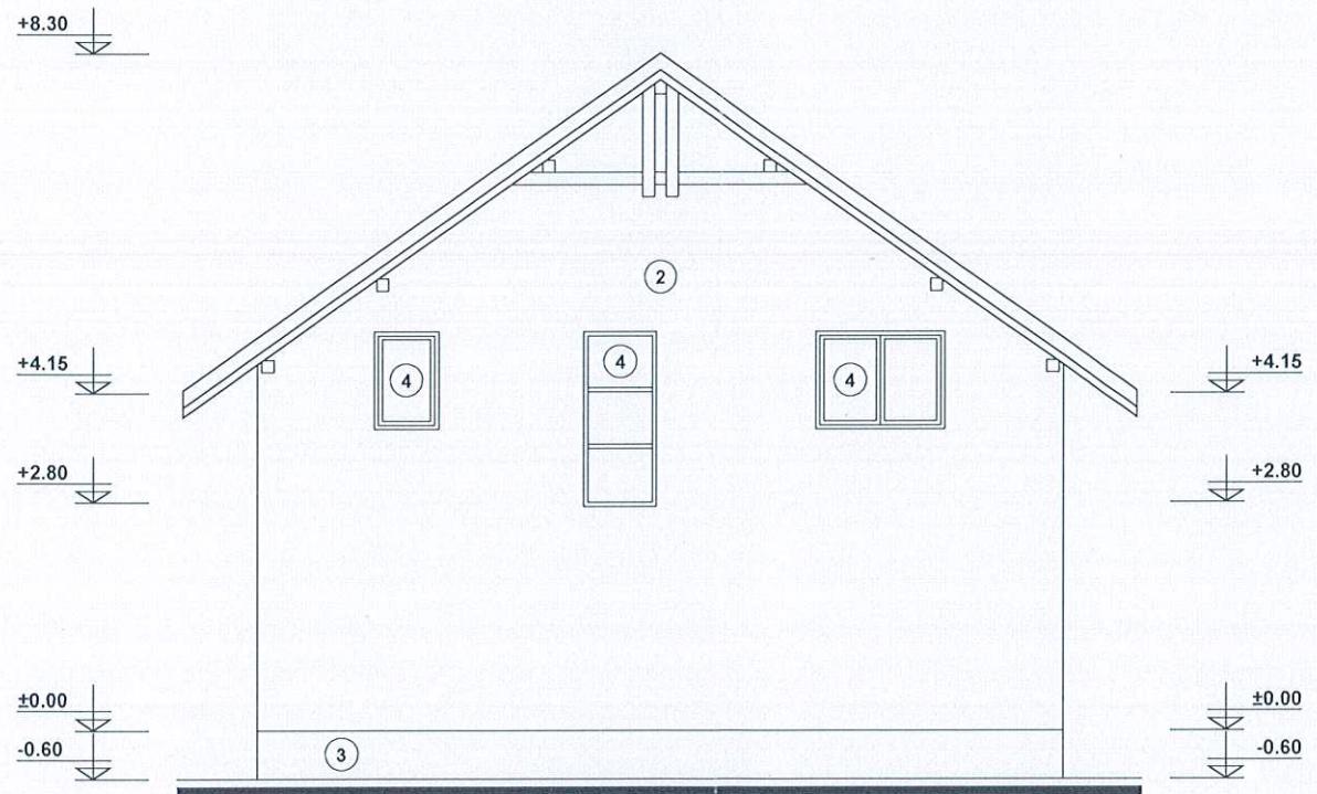
FATADA POSTERIOARA Scara 1:100
